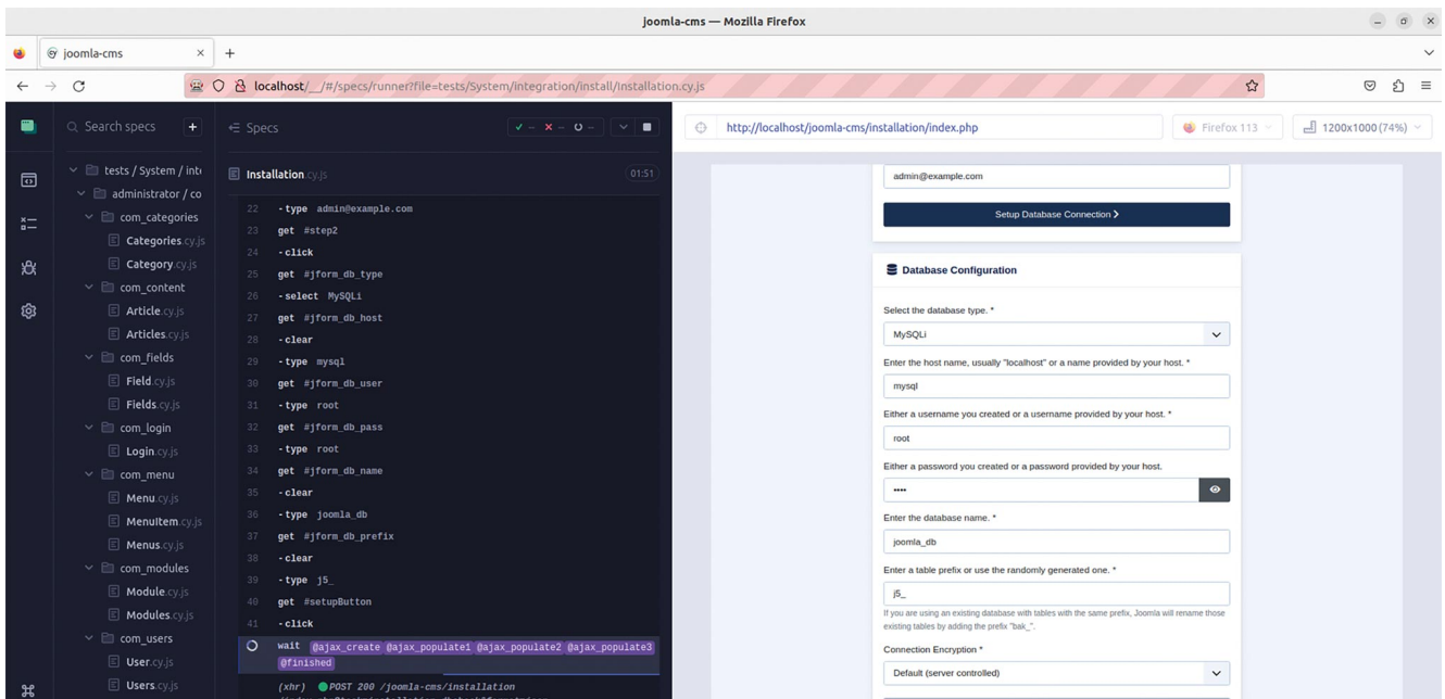
Abb. 10: Der Test, der die korrekte Installation von Joomla! sicherstellt, während der Ausführung
