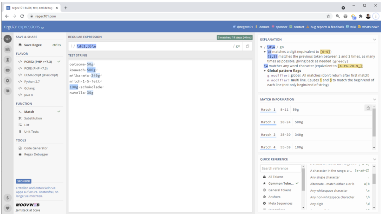
Abbildung 5: In diesem Beispiel wurde nach 1 bis 3 aufeinanderfolgenden Ziffern gesucht – und zusätzlich definiert, dass direkt hinter der Ziffer ein Buchstabe kommen muss
